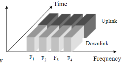
FDMA/TDD
