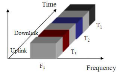
TDMA/TDD
