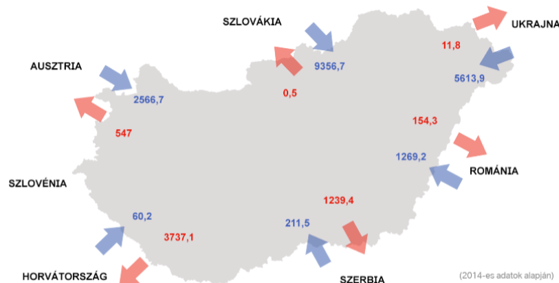
A határkeresztező távvezetéseken ténylegesen mért villamosenergia-forgalom
