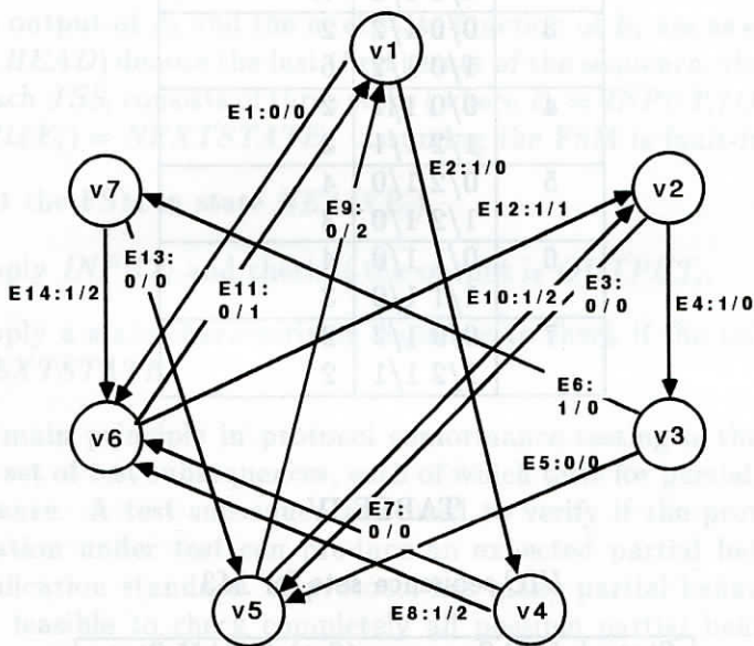
Fig. 17. A sample FSM ( M3 ) – dk27
